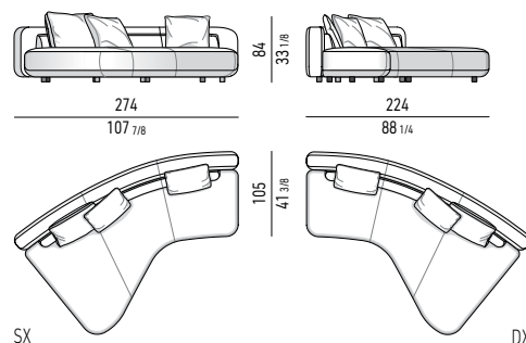
ELEMENTO CENTRALE CM 274X224 - DOPPIA PROFONDITÀ CENTRAL ELEMENT CM 274X224 - DOUBLE DEPTH
