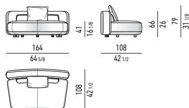
ELEMENTO CENTRALE CM 164 CENTRAL ELEMENT CM 164
