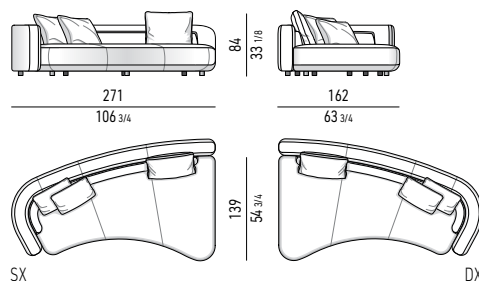
ELEMENTO TERMINALE CM 271X162 - DOPPIA PROFONDITÀ ELEMENT WITH 1 ARMREST CM 271X162 - DOUBLE DEPTH
