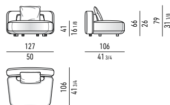
ELEMENTO CENTRALE CM 127 CENTRAL ELEMENT CM 127
